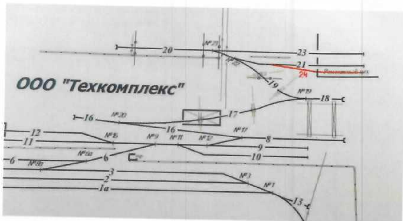
Примыкание пути «№24»
